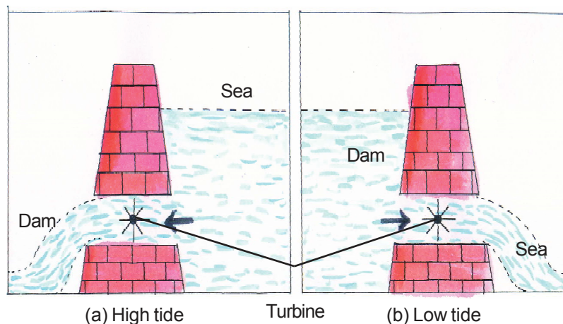
Fig 12.3 Tidal energy
