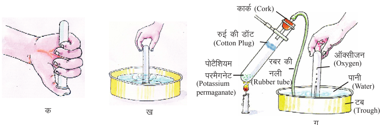
चित्र 3.1 ऑक्सीजन गैस बनाना (Preparation of Oxygen Gas)
