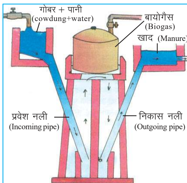
चित्र 12.9 बायो गैस संयंत्र (Bio-gas plant)
