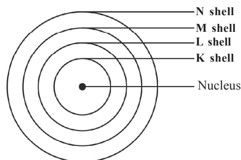
Fig. 6 : Atomic shells
