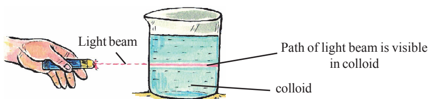
Fig. 5 : Tyndall effect
